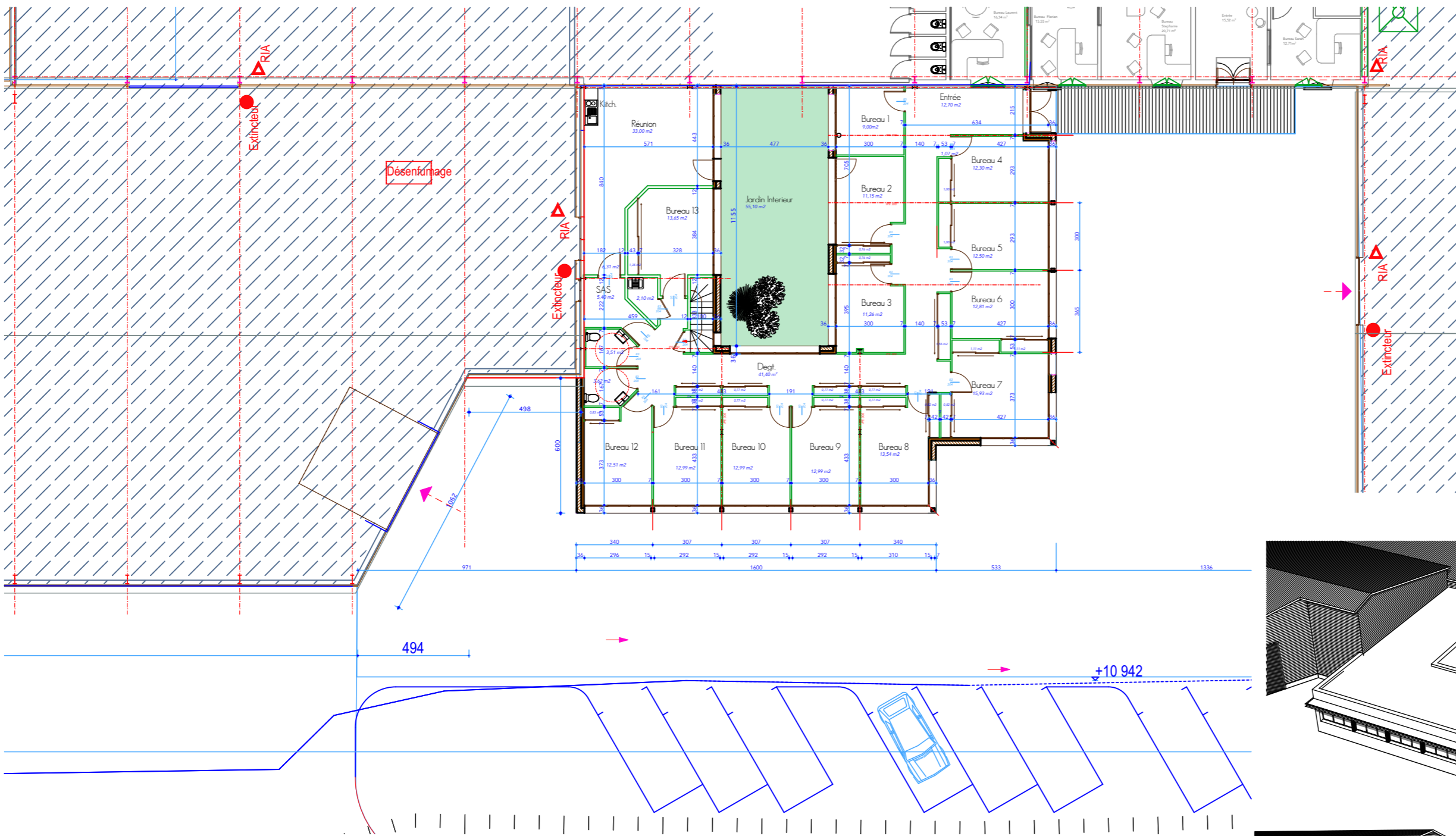
Plan des Bureaux Ech: 1/200
